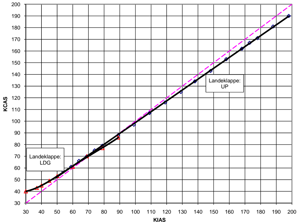
Abb.: 5.2.1 Fahrtmesserkorrektur
