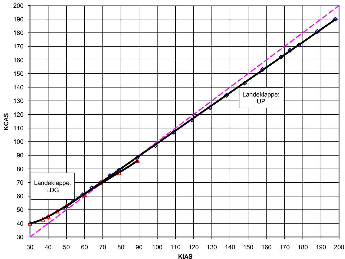
Abb.: 5.2.1 Fahrtmesserkorrektur
