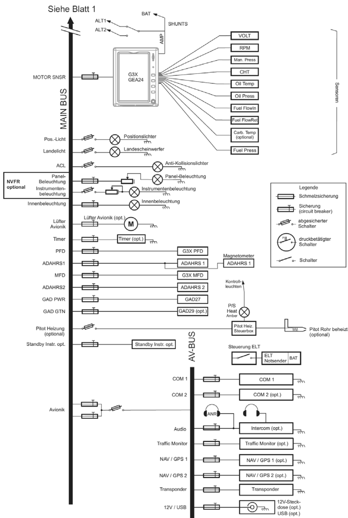
Abb.: Blockschaltbild Elektrik 2/2 (G3X-Version)
