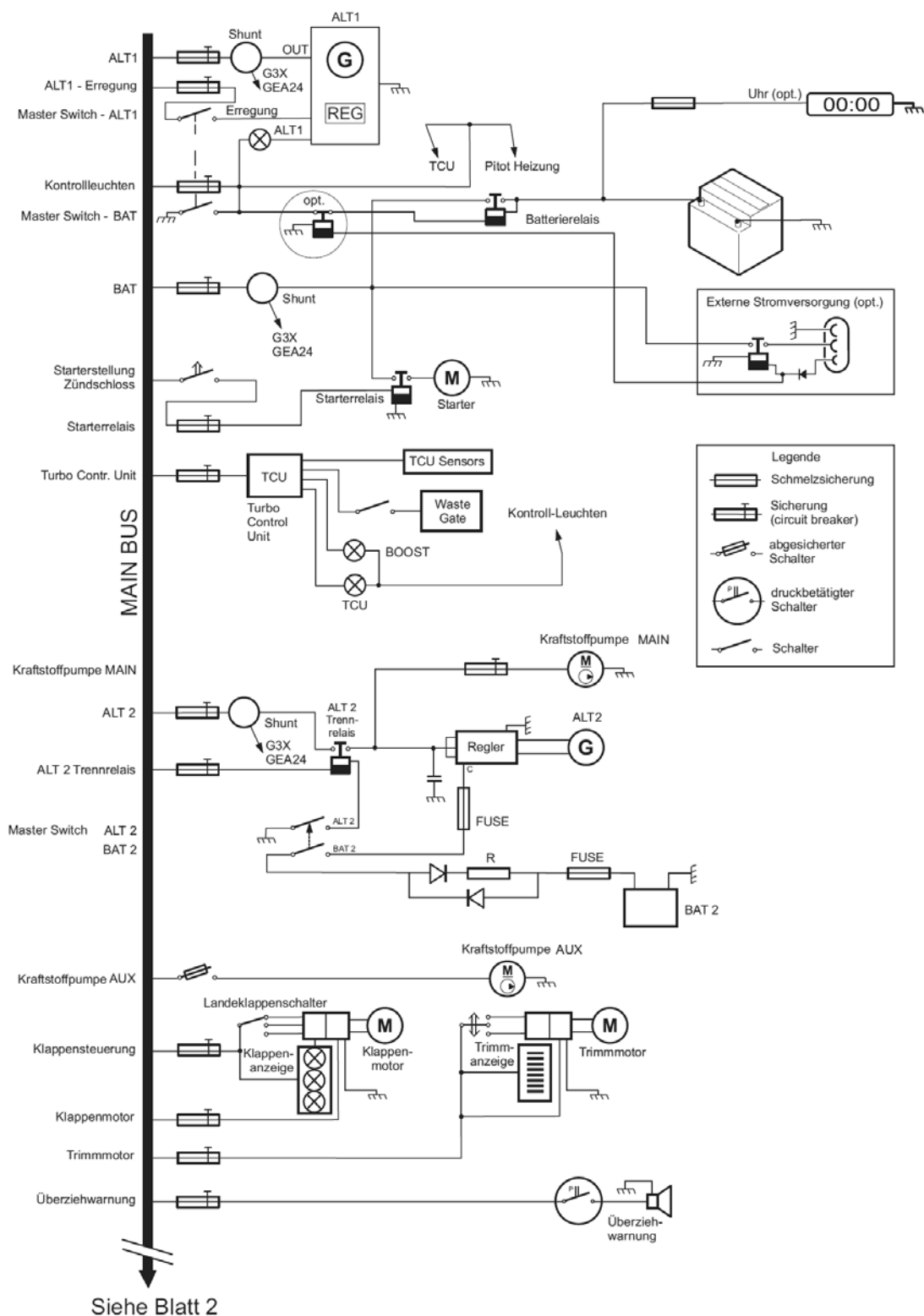
Abb.: Blockschaltbild Elektrik 1/2 (G3X-Version)
