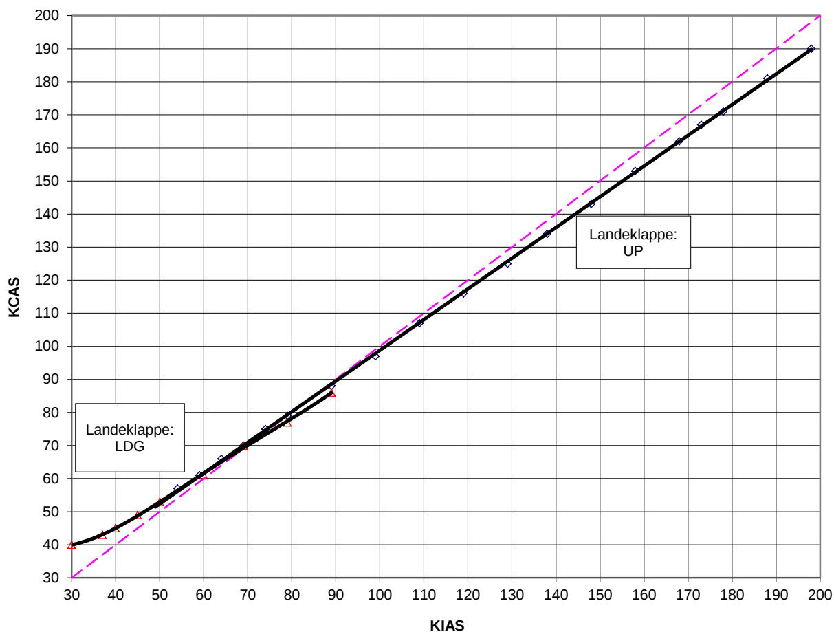
Abb.: 5.2.1 Fahrtmesserkorrektur
